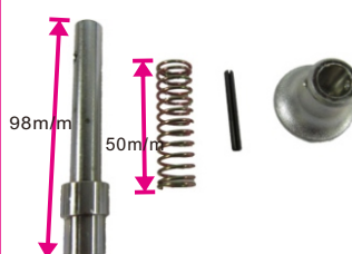
TOYOTA 5FD45 12*98m/m (彈簧50m/m)
