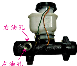
右油孔 左油孔 46010-35H10 NISSAN FB15 (電動車) 1-1/16" NI-104-1
